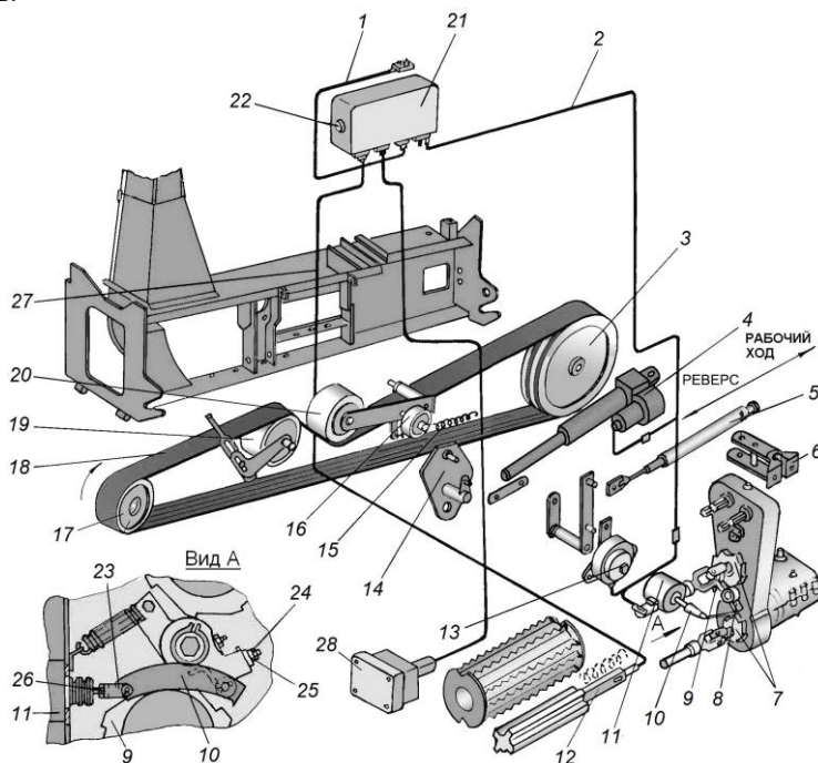
Рис. 22. Система защиты рабочих органов: 1 – жгут входной; 2 – жгут выходной; 3 – шкив ведомый; 4 – исполнительный электромеханизм; 5 – тяга переключателя реверса; 6 – рычаг реверса; 7 – храповые механизмы; 8 – собачка; 9, 15 – пружины; 10 – тяга; 11 – электромагнит основания; 12 – датчик металлодетектора; 13 – датчик положения; 14 – фигурный рычаг; 16 – упорный ролик; 17 – ведущий шкив; 18 – ремень; 19 – обводной ролик; 20 – натяжной ролик; 21 – электронный блок; 22 – переключатель уровня чувствительности; 23 – вилка; 24, 26 – контргайки; 25 – гайка; 27 – жгут датчика металлодетектора; 28 – датчик камнедетектора
