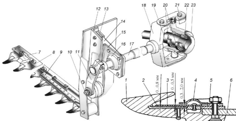
Рис. 7. Механизм «качающейся шайбы»:
