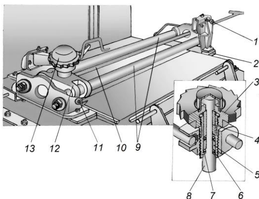
Рис. 5. Заточное приспособление:
