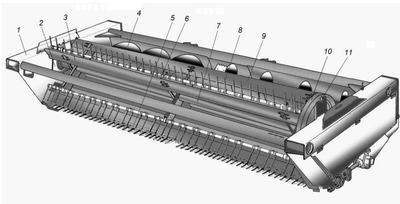
Рис. 6. Жатка для трав: 1 – рама; 2 – опора мотовила; 3 – мотовило; 4 – шнек; 5 – режущий аппарат; 6 – граблина; 7 – вал мотовила; 8 – пружинный зуб; 9 – планка мотовила; 10 – направляющая дорожка; 11 – монтажное окно
