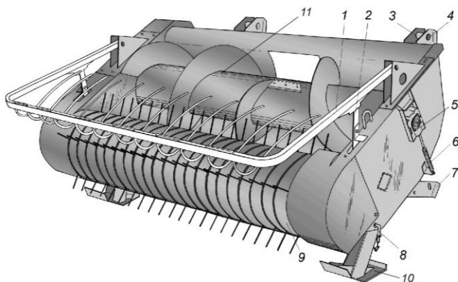
Рис. 9. Подборщик:
