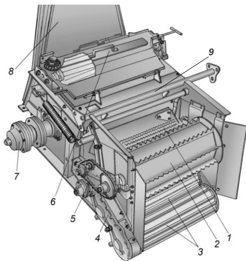
Рис. 3. Питающий аппарат:
