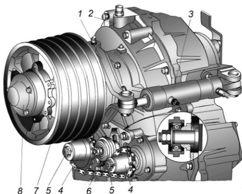
Рис. 11. Привод питающего аппарата:
