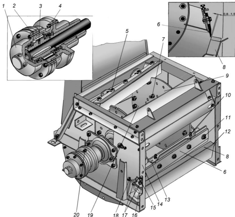
Рис. 4. Измельчающий аппарат: 1 – крышка обгонной муфты; 2 – пружина; 3 – шарик; 4 – корпус; 5 – болт крепления ножа; 6 – нож; 7 – болт крепления опоры ножа; 8 – противорежущий брус; 9 – диск; 10 – установочный винт; 11 – прижим ножа; 12 – чистик; 13 – опора ножа; 14 – рама; 15 – прижимной болт; 16 – прижим; 17 – контргайка; 18 – регулировочный болт; 19 – барабан; 20 – предохранительный болт
