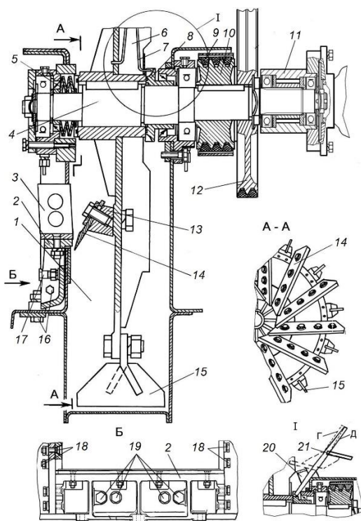
Рис. 16. Измельчающий аппарат:
