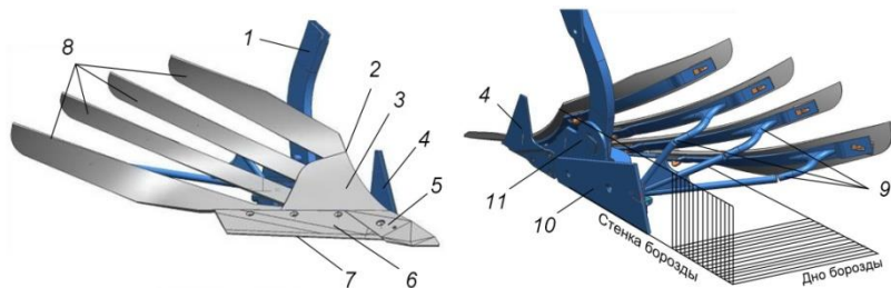
Рис. 2. Корпус плуга в сборе со стойкой: 1 – стойка; 2 – полевой обрез; 3 – грудь отвала; 4 – нож полевой доски; 5 – долото; 6 – лемех; 7 – лезвие лемеха; 8 – пластины отвала; 9 – распорки; 10 – полевая доска; 11 – башмак
