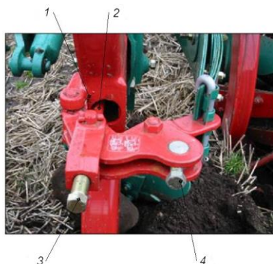
Рис. 11. Регулировка предохранителя: 1 – труба; 2 – тяга; 3, 4 – болты
