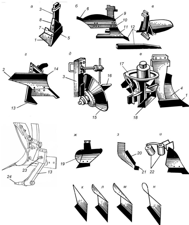
Рис. 3. Корпуса плугов: а – безотвальный; б – вырезной; в – с выдвигаемым долотом; г – с почвоуглубителем; д – дисковый; е – комбинированный; ж – для ромбической вспашки; з – чизельный; и – роликовый; к, л, м, н – типы корпусов; 1, 10 и 11 – лемеха; 2 и 9 – отвалы; 3 – стойка корпуса; 4 – грудь отвала; 5 – полевая доска; 6 – перо отвала; 7 – уширитель; 8 – щиток; 12 – долото; 13 – почвоуглубитель; 14 – углосним; 15 – диск; 16 – чистик; 17 – ротор; 18 – лопатки; 19 – боковой отвал; 20 – обтекатель; 21 – долото; 22 – ролик; 23 – держатель; 24 – сменное острие
