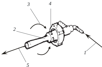
Рис. 5. Гидравлическая мешалка 1, 3, 5 – потоки жидкости; 2 – дроссель; 4 – отверстия
