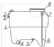
Рис. 3. Бак опрыскивателя: 1 – бак основной; 2 – бак дополнительный; 3 – кран для мытья рук; 4 – гидромешалка; 5 – заборный патрубок (антиворонка); 6 – уровень; 7 – фильтр корзиновый; 8 – заливная горловина
