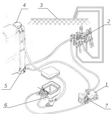
Рис. 11. Схема жидкостной системы опрыскивателя «JACTO FALCON AM-14»:
