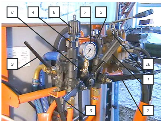
Рис. 13. Пульт управления: 1 – переключатель «работа-заправка»; 2, 3 – рукоятки включения подачи жидкости на секции штанги; 4, 5 – регуляторы секций штанги; 6 – основной регулятор давления; 7 – манометр; 8 – кран манометра; 9 – кран включения мешалки; 10 – гидрораспределитель
