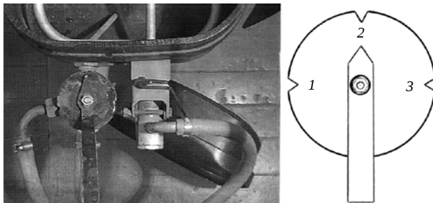
Рис. 15. Кран управления работой смесителя и возможные положения
