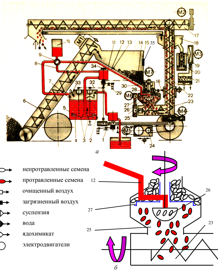
Рис. 7. Протравливатель ПС-10: а – технологическая схема работы; б – схема технологического процесса работы камеры протравливания; 1 – заправочный насос; 2, 7, 13, 14, 30, 35 – датчики; 3 – мешалки; 4 – резервуар; 5 – электронагреватель; 6 – загрузочный транспортер; 8, 12 – трубопроводы; 9 – кран; 10 – мерный цилиндр; 11 – насос-дозатор; 15 – бункер; 16 – рычаг дозатора подачи семян; 17, 22, 23 – шнековые транспортеры выгрузки; 18 – воздуховод с коллектором; 19 – вентилятор; 20 – камера фильтрации; 21 – фильтр; 24 – передача самохода; 25 – камера протравливания; 26 – распылитель; 27 – семенной диск; 28 – распределитель; 29 – электромагнит; 31, 32 – цепные передачи; 33 – горловина; 34 – регулятор дозатора
