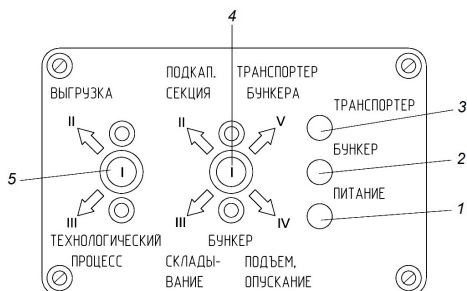
Рис. 12. Пульт управления гидросистемой комбайна: 1, 2, 3 – светодиоды; 4, 5 – переключатели
