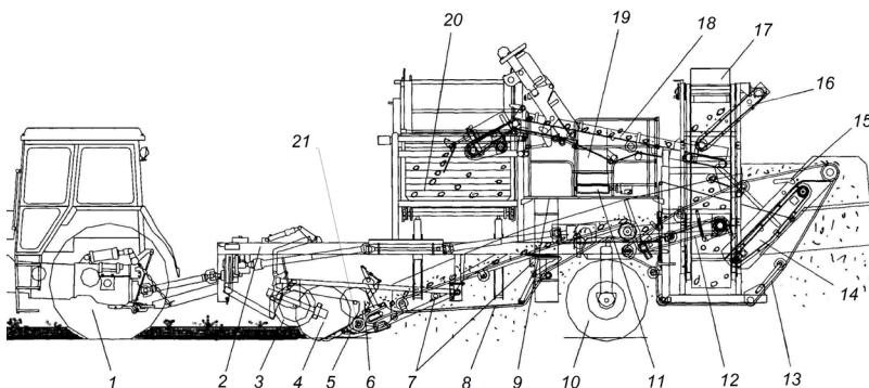
Рис. 8. Схема технологического процесса работы комбайна ПКК-2-02:
