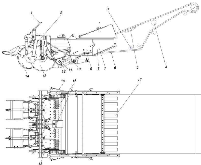
Рис. 9. Подкапывающе-сепарирующий блок:
