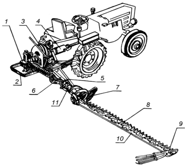
Рис. 1. Общий вид косилки КС-2,1:
