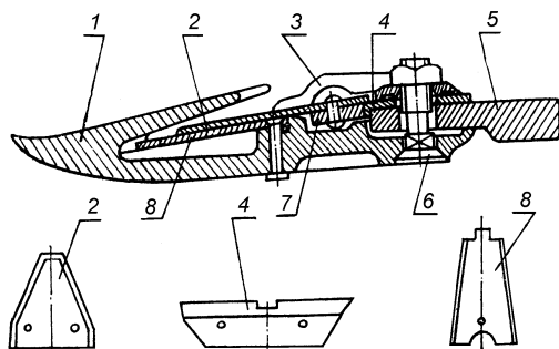
Рис. 2. Режущий аппарат косилки КС-2,1:
