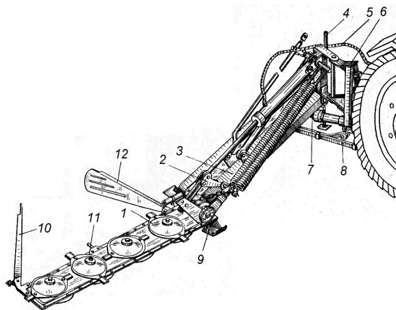
Рис. 8. Общий вид косилки КДН-210:
