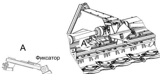
Рис. 16. Изменение режима продольного копирования
