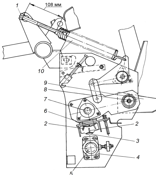
Рис. 7. Схема регулирования плющильного аппарата: 1 – болт; 2 – ребро; 3 – нижний валец; 4 – корпус; 5, 7 – карданные валы; 6 – верхний валец; 8 – болт; 9 – боковой щиток; 10 – пружина
