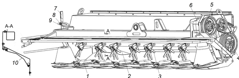
Рис. 12. Боковая секция:
