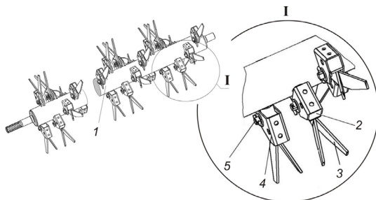
Рис. 14. Ротор плющильного аппарата: 1 – вал; 2 – демпфер; 3 – бич; 4 – корпус; 5 – ось со шплинтом
