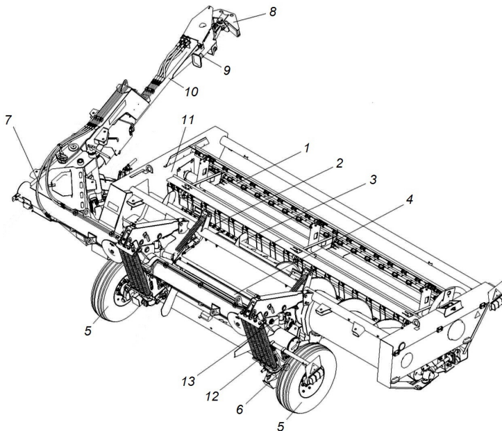
Рис. 3. Косилка-плющилка прицепная КПП-4,2:
