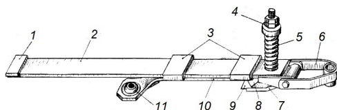
Рис. 10. Тяговый предохранитель косилки КДН-210:
