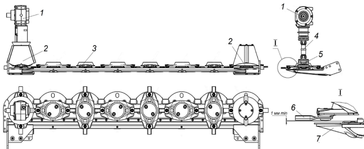
Рис. 13. Режущий брус:
