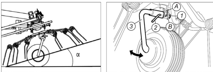
Рис. 11. Схема к настройке угла разбрасывания:
