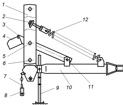
Рис. 5. Система подвески граблей: 1 – стойка; 2 – регулировочный винт; 3 – упор; 4 – защелка; 5 – палец; 6 – шкворень; 7 – подвесная цепь; 8 – пружина; 9 – опора; 10 – стрела рамы; 11 – ось; 12 – пружина
