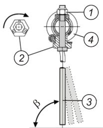
Рис. 12. Схема к настройке вертикального положения зубьев ротора: 1 – крепежная гайка; 2 – эксцентриковая втулка; 3 – зуб; 4 – труба ротора
