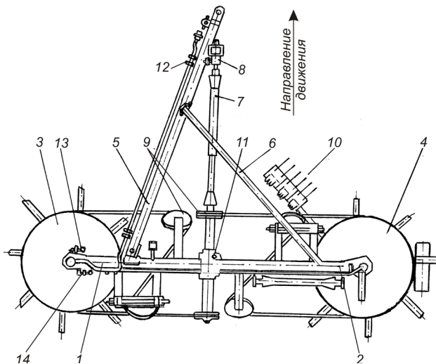
Рис. 1. Схема граблей ГВР-630 (рабочее положение):
