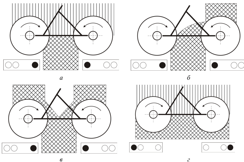
Рис. 3. Варианты установки копиров при выполнении технологических операций: а – сгребание; б – оборачивание вала; в – сдвигание валков; г – ворошение; ● ○ ○ – положение фиксатора рукоятки копира
