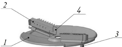
Рис. 4. Метатель (рассеивающий диск): 1 – диск; 2 – лопатка; 3 – фиксатор; 4 – направляющая
