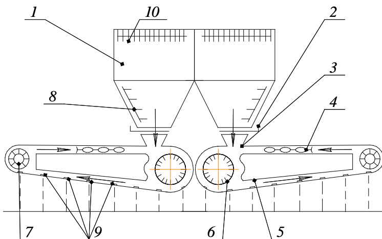
Рис. 14. Схема подкормщика РШУ-12: 1 – бункер; 2 – заслонка; 3 – приемный лоток; 4 – цепь с шайбами; 5 – распределительная штанга; 6 – ведущий шкив; 7 – ведомый шкив; 8 – ворошитель; 9 – высевные отверстия; 10 – сетка
