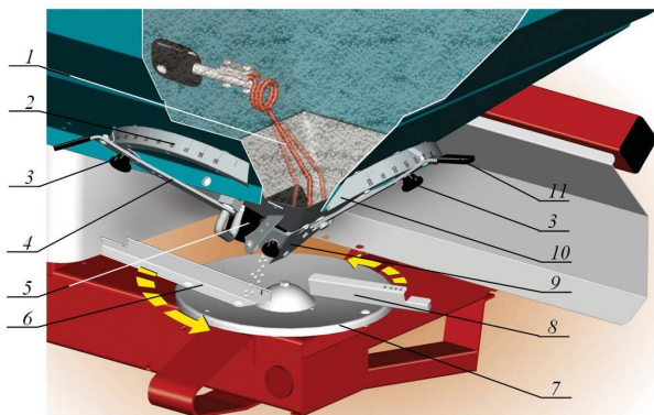
Рис. 8. Рассеивающий узел:
