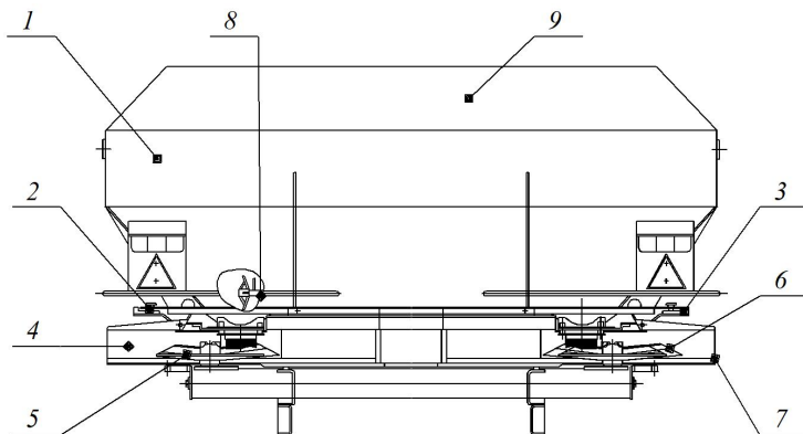
Рис. 2. Общий вид рассеивателя PY-1600: 1 – бункер с рамой; 2 – механизм дозирующий правый; 3 – механизм дозирующий левый; 4 – отражатель правый; 5 – метатель (рассеивающий диск) правый; 6 – метатель (рассеивающий диск) левый; 7 – отражатель левый; 8 – рыхлитель (сводоразрушитель); 9 – тент
