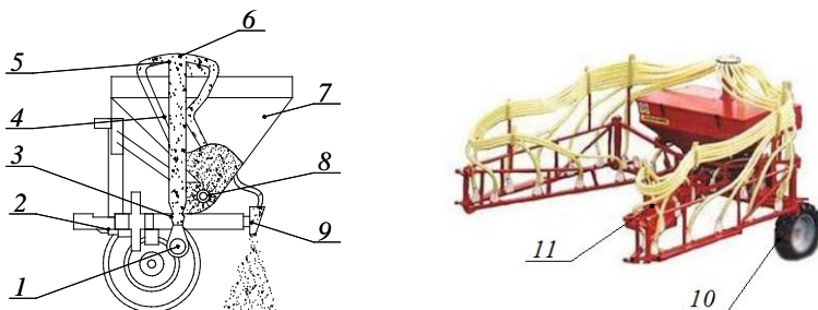
Рис. 13. Технологическая схема пневматической штанговой сеялки СУ-12:
